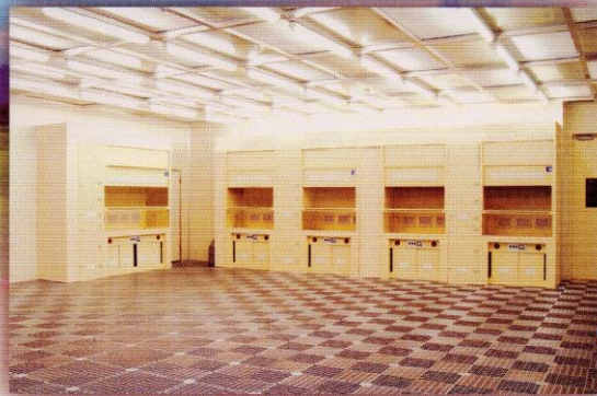
●ドラフトチャンバー設置例
