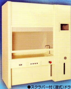
●スクラバー付(湿式)ドラフトチャンバー
