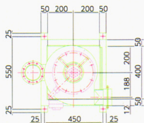
スーパー・クリーン SK-3型 (湿式、乾式併用式)
