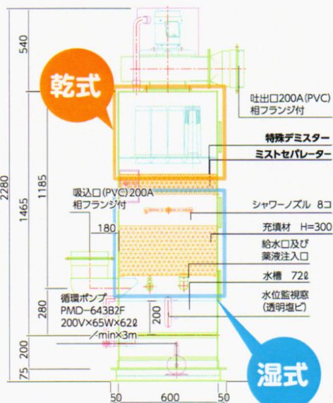
スーパー・クリーン SK-20型(20m 3 /min)
