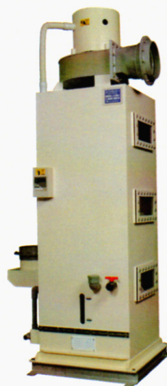
スーパー・クリーン SK-20型(20m 3 /min)
