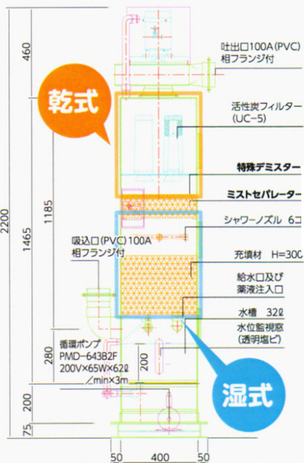
スーパー・クリーン SK-3型(3m 3 /min)
