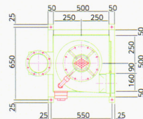
スーパー・クリーン SK-10型 (湿式、乾式併用式)
