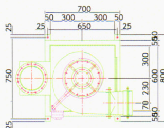
スーパー・クリーン SK-10型(10m 3 /min)
