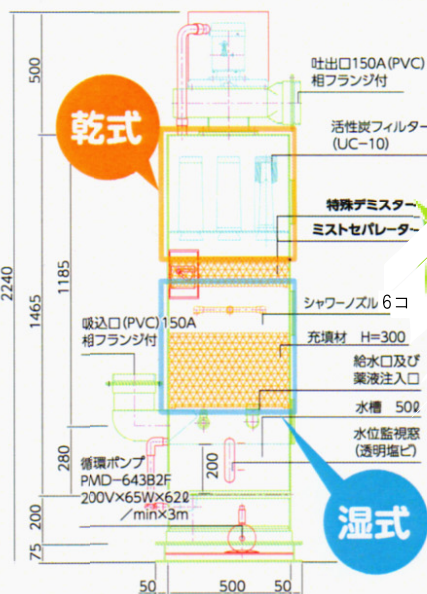
スーパー・クリーン SK-10型(10m 3 /min)
